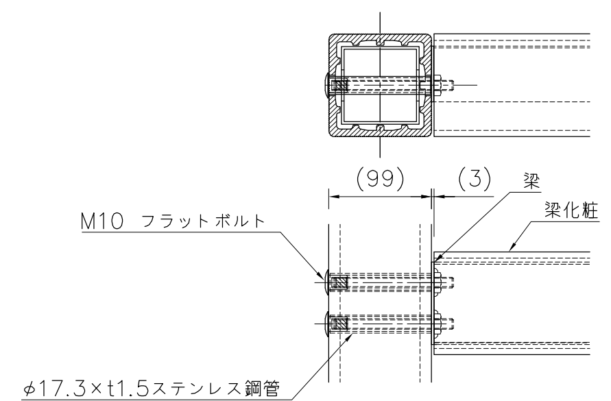
A部詳細 S=1/5
