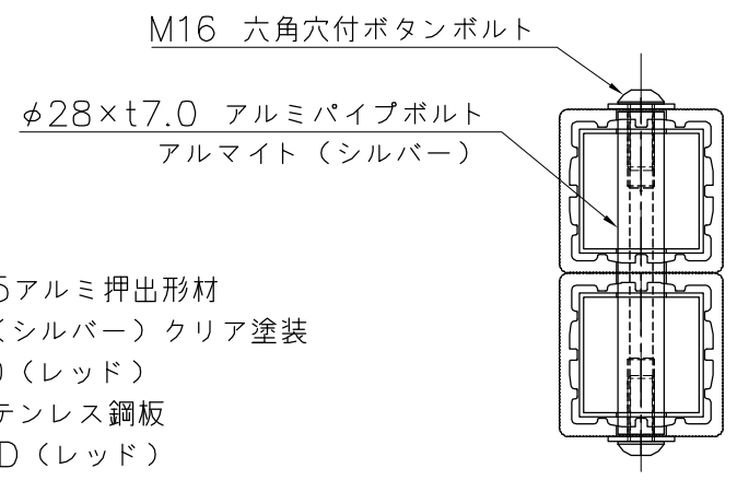
C部詳細 S=1/5
