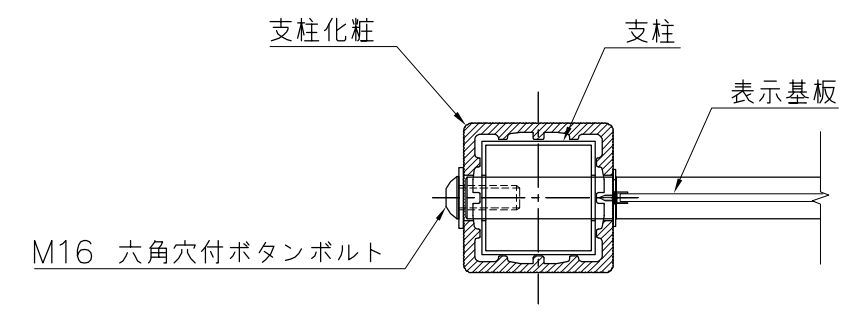
B部詳細 S=1/5
