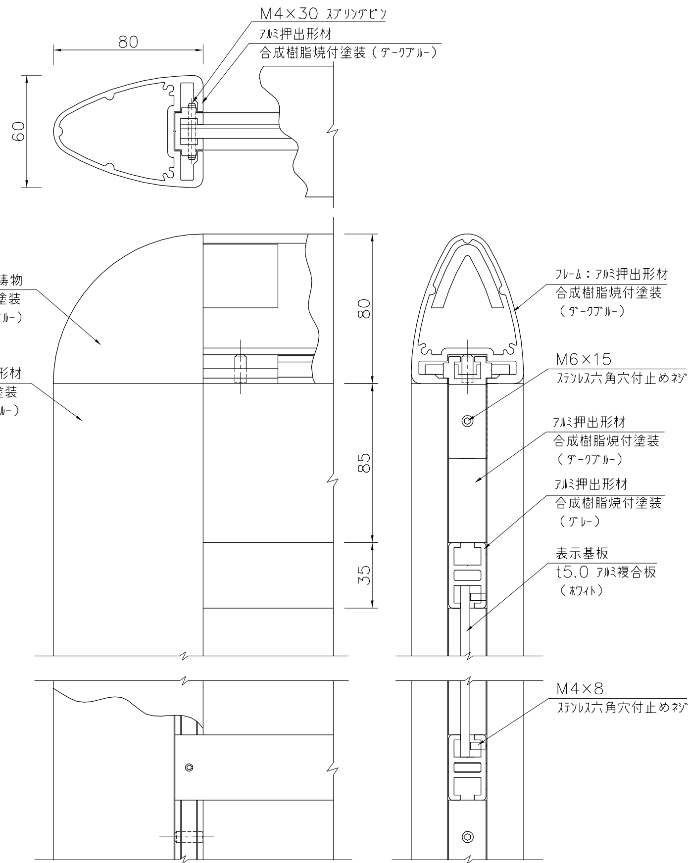
詳細図 S=1/2
