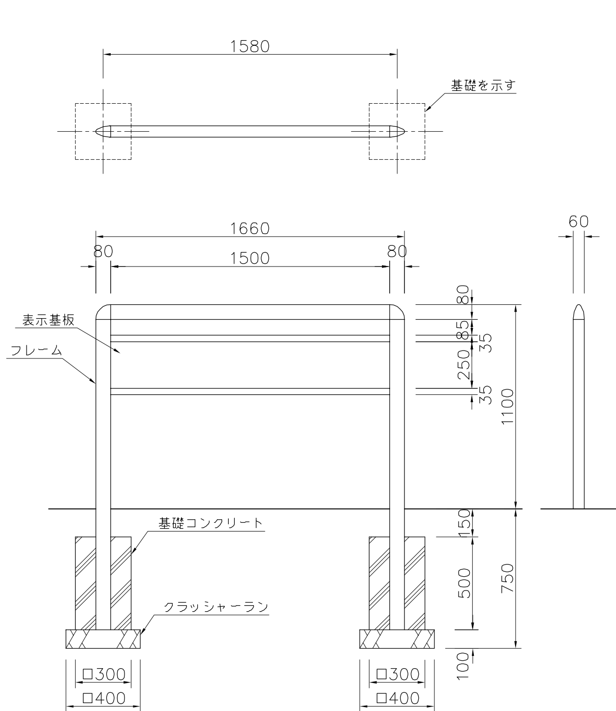
外観図 S=1/20
