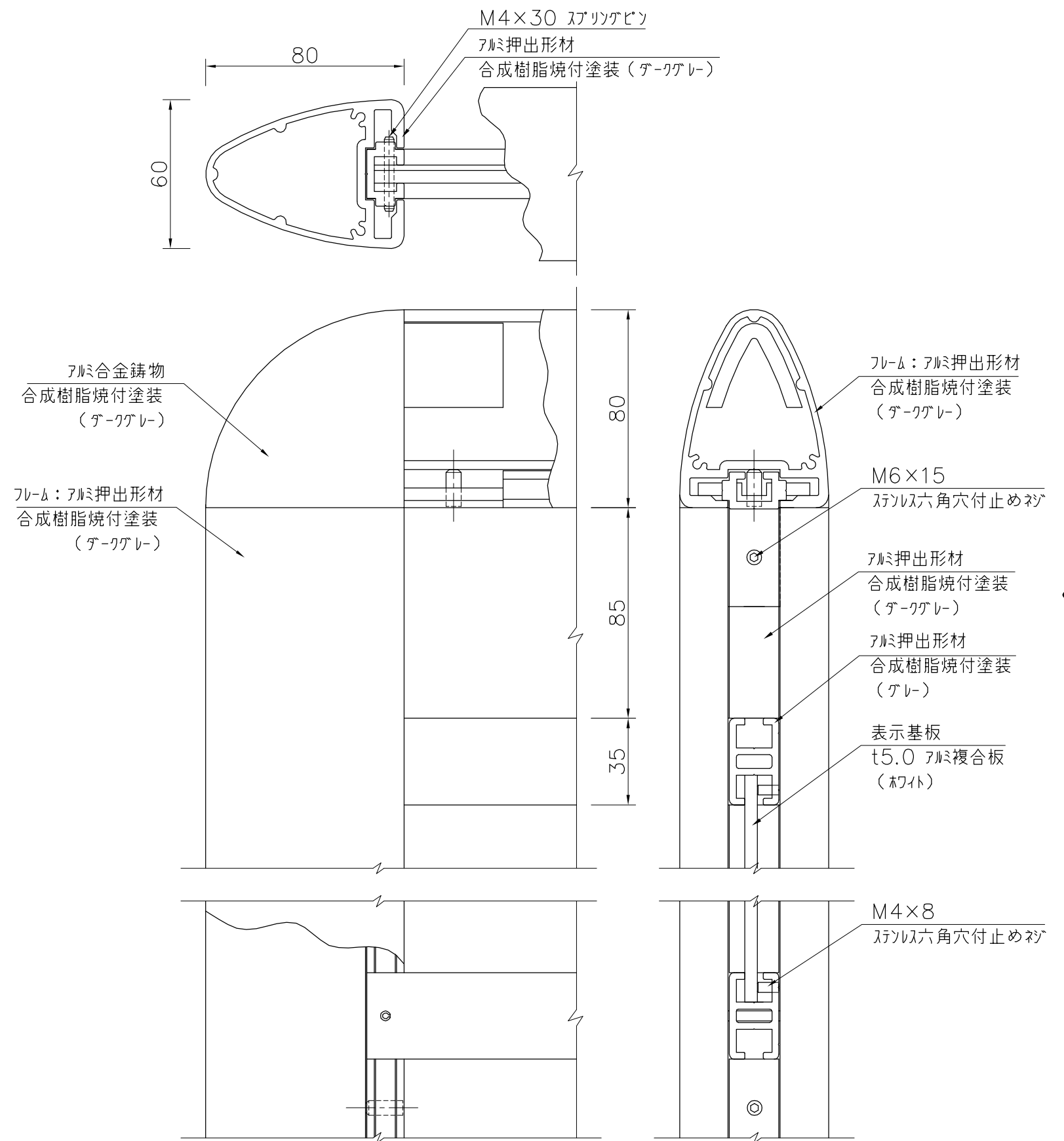
詳細図 S=1/2
