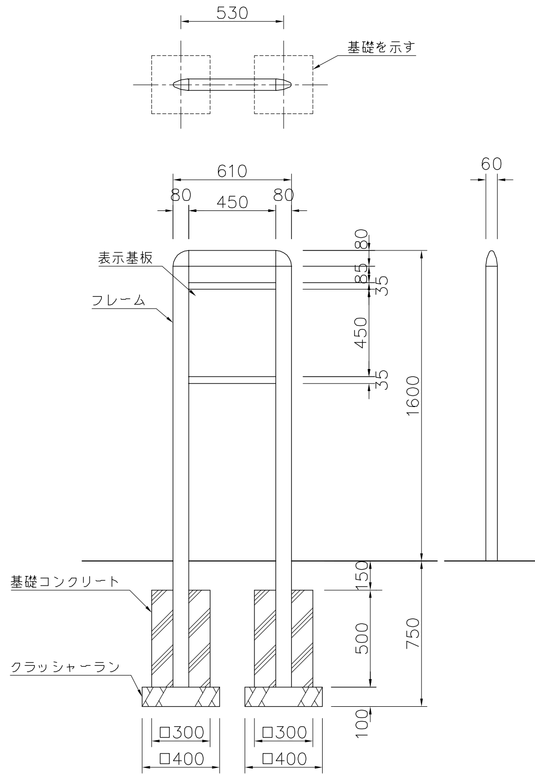
外観図 S=1/20
