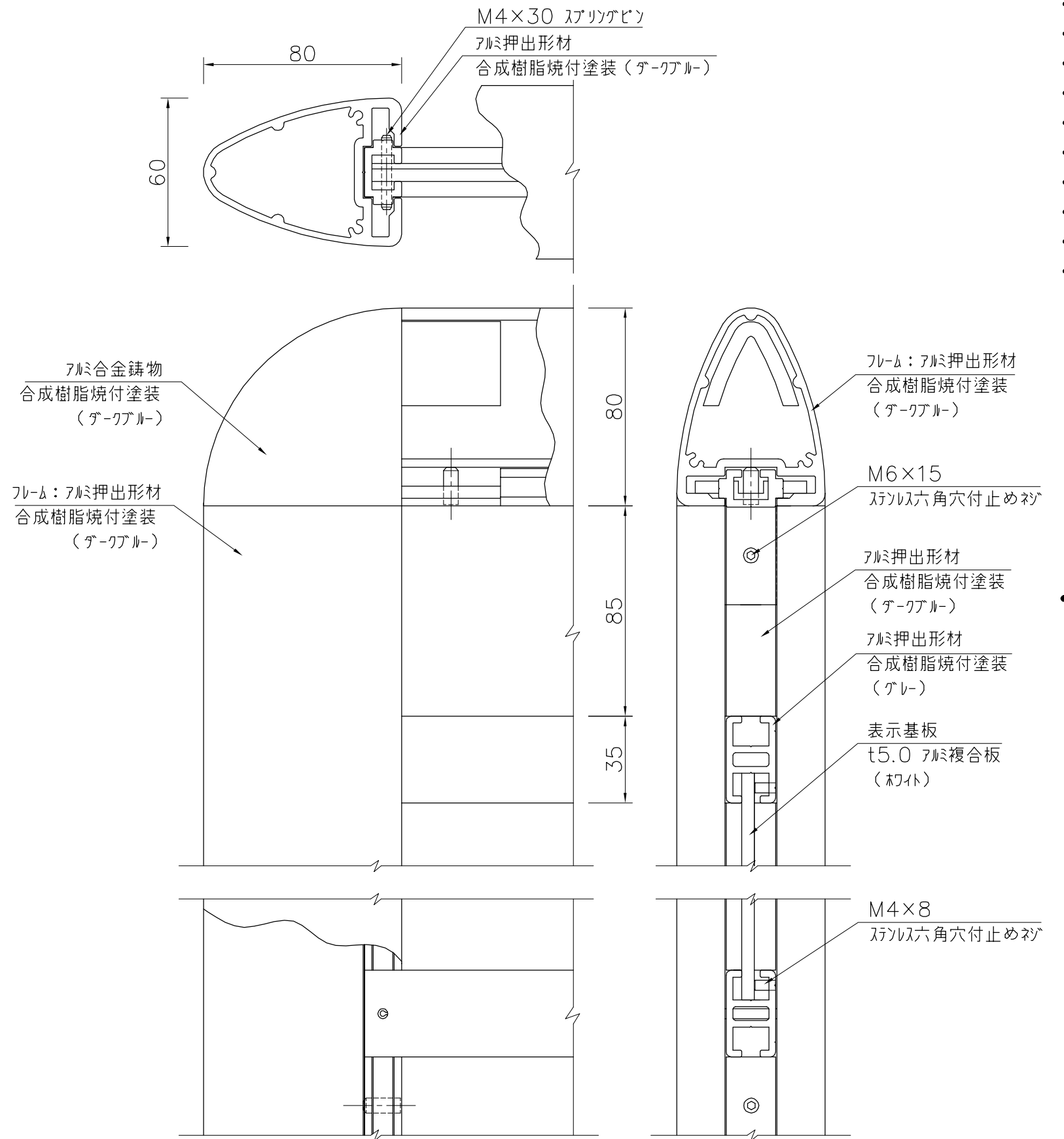
詳細図 S=1/2
