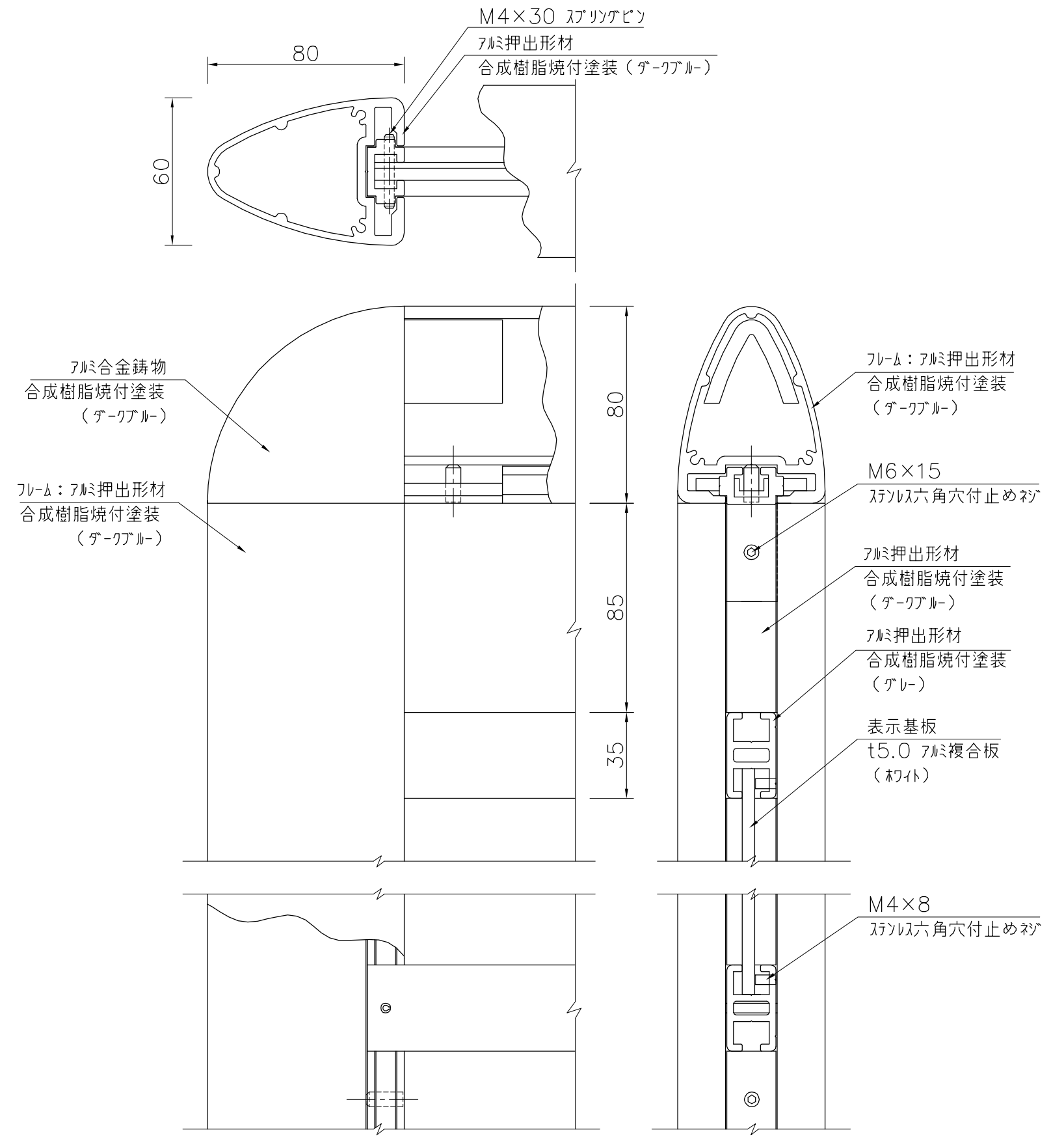
詳細図 S=1/2
