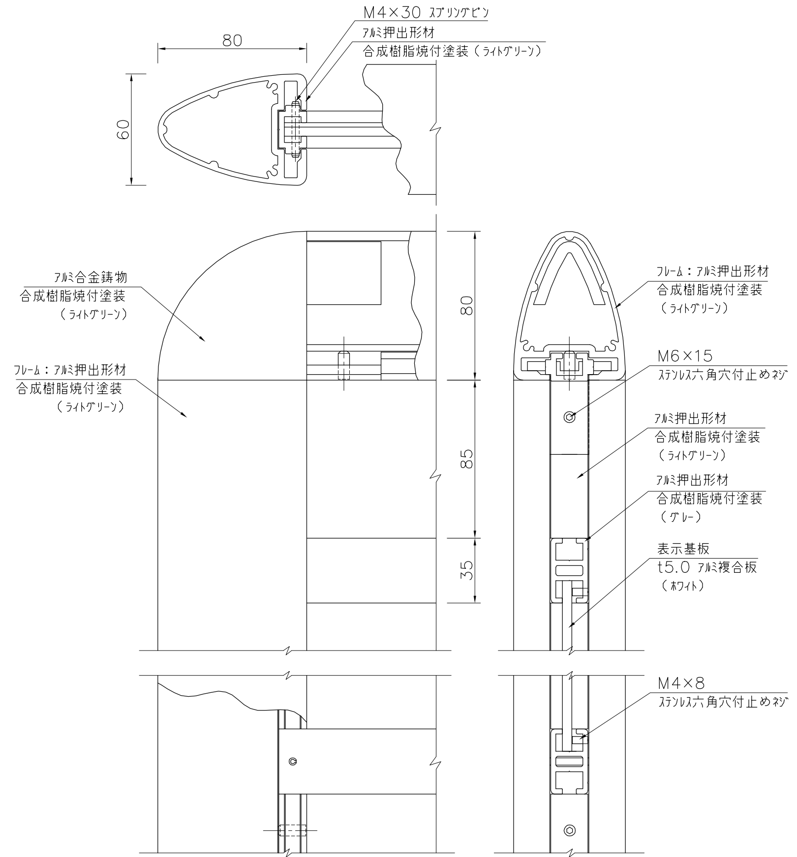
詳細図 S=1/2
