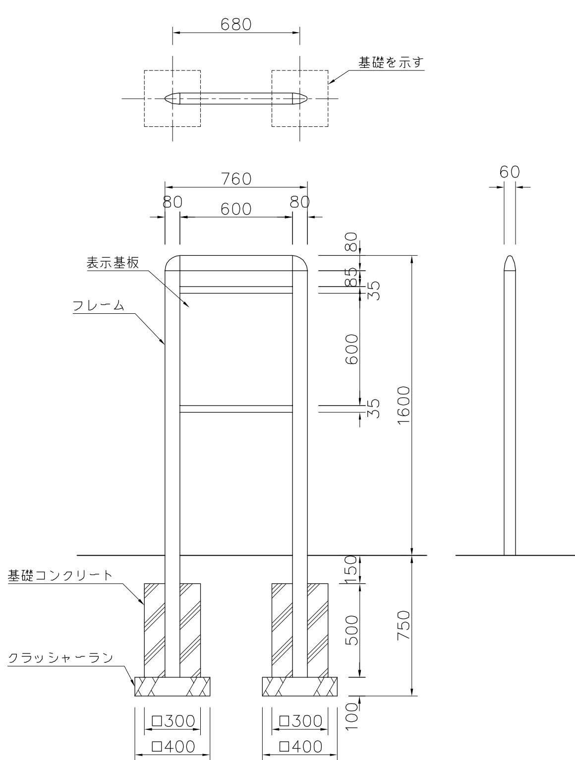
外観図 S=1/20
