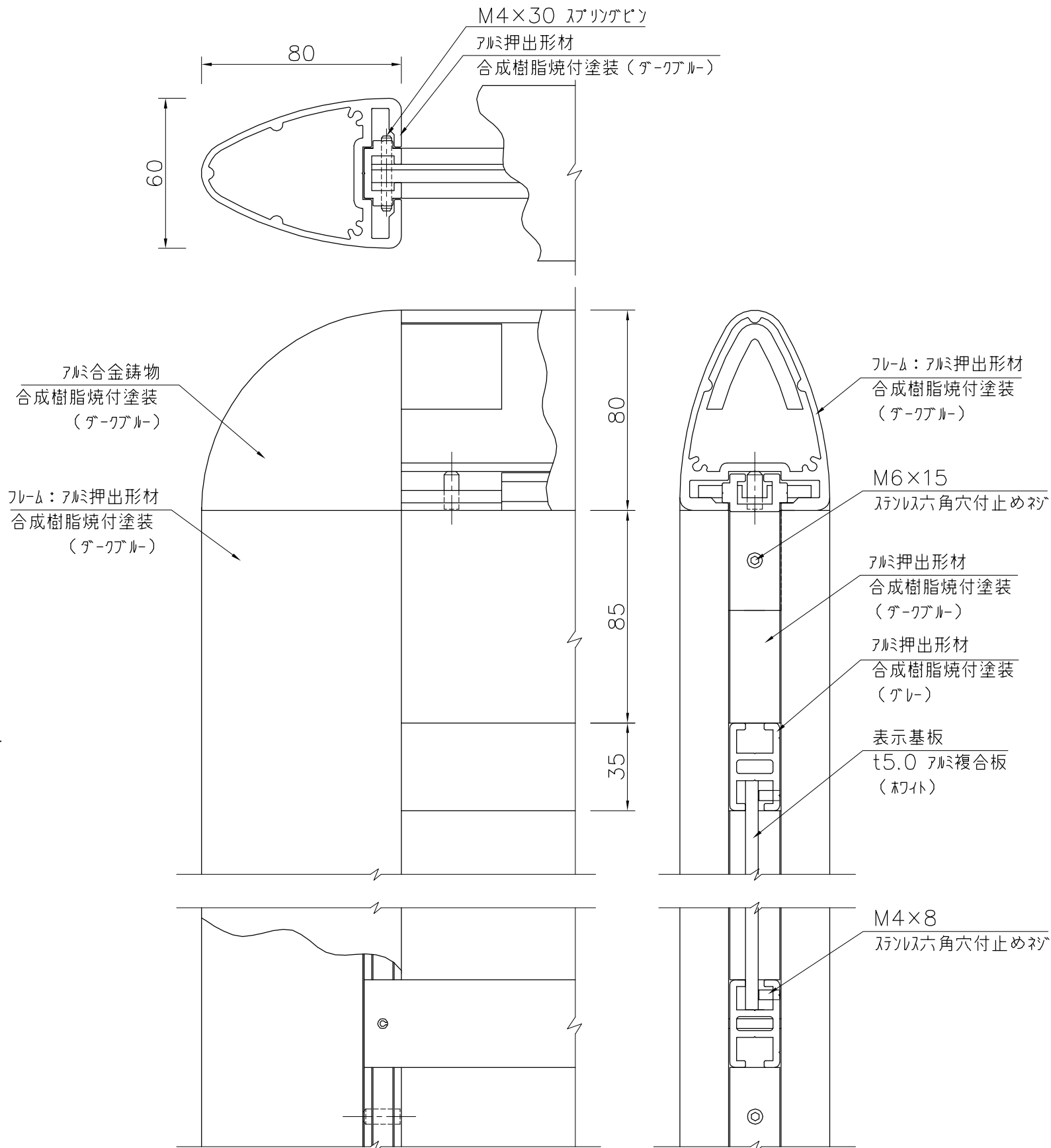
詳細図 S=1/2
