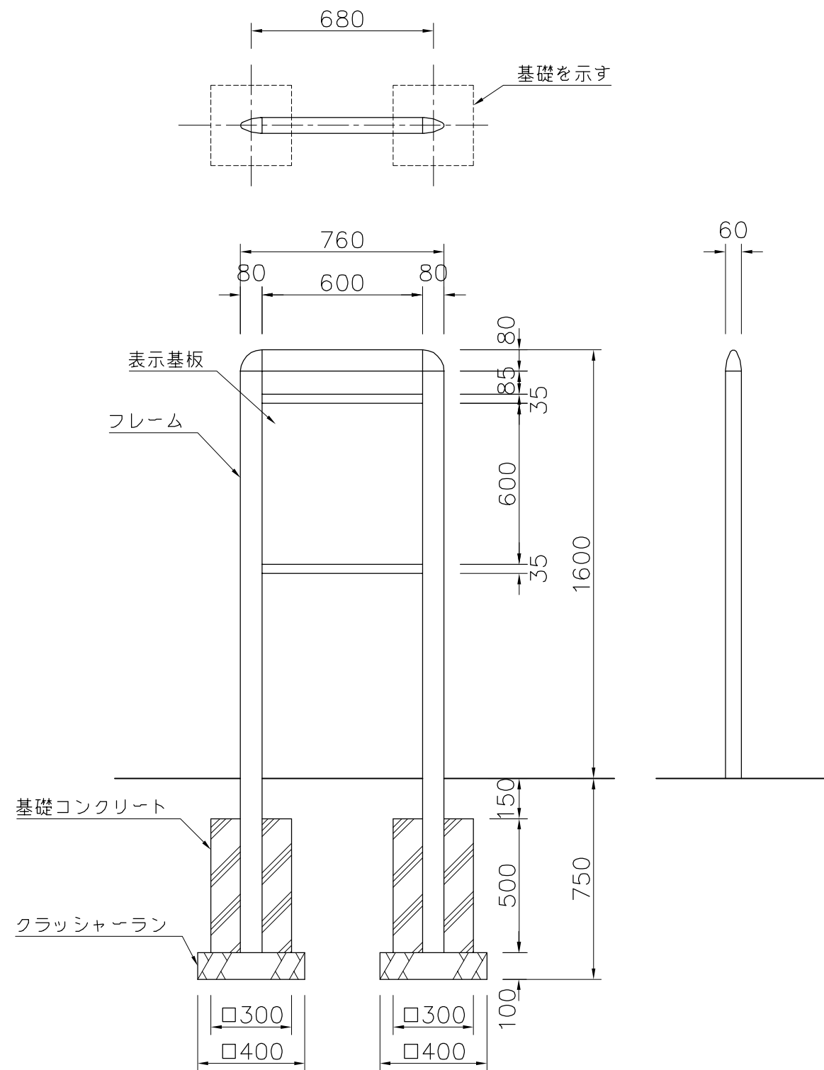
外観図 S=1/20
