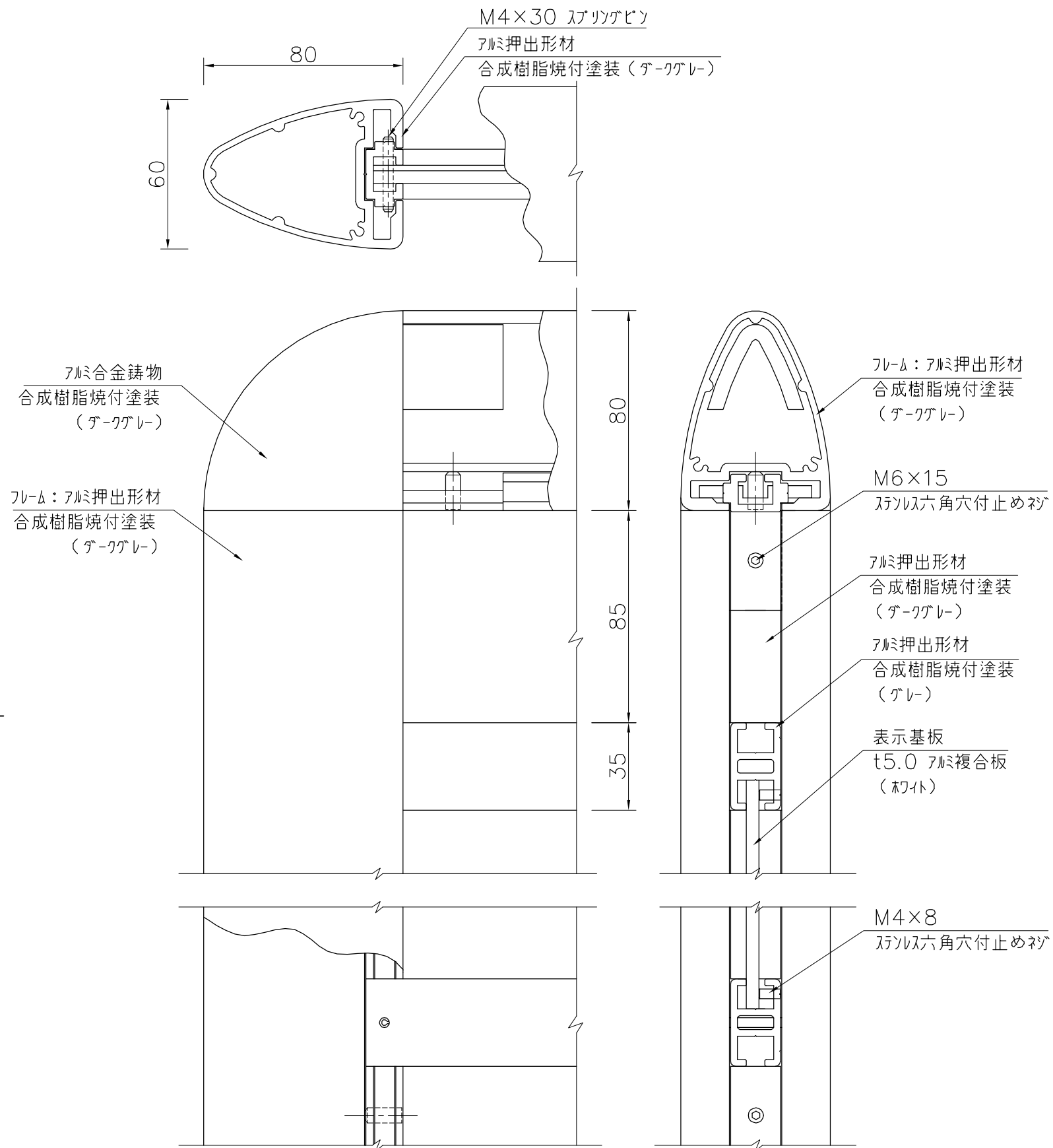
詳細図 S=1/2
