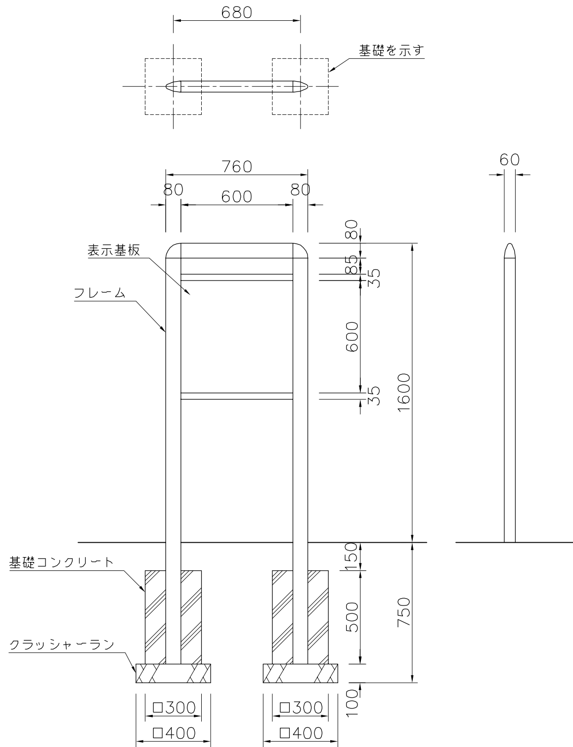
外観図 S=1/20
