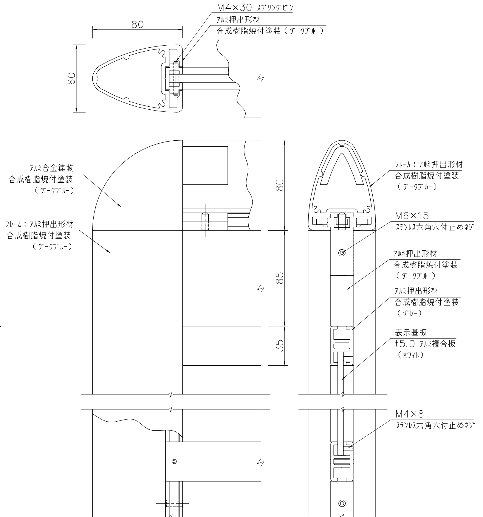
詳細図 S=1/2
