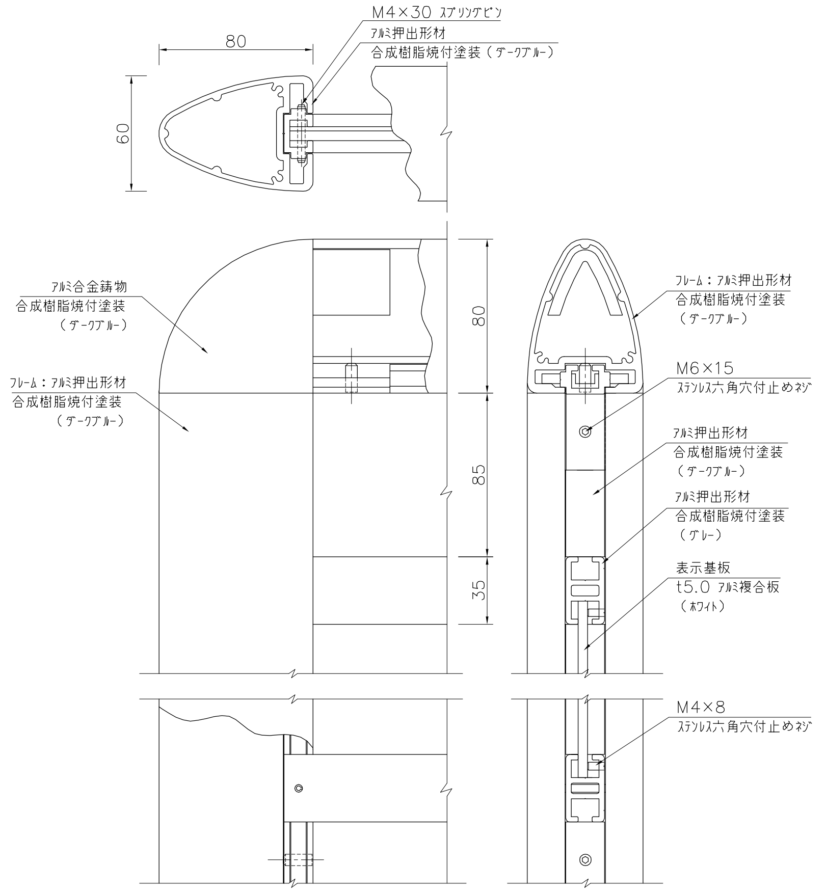
詳細図 S=1/2
