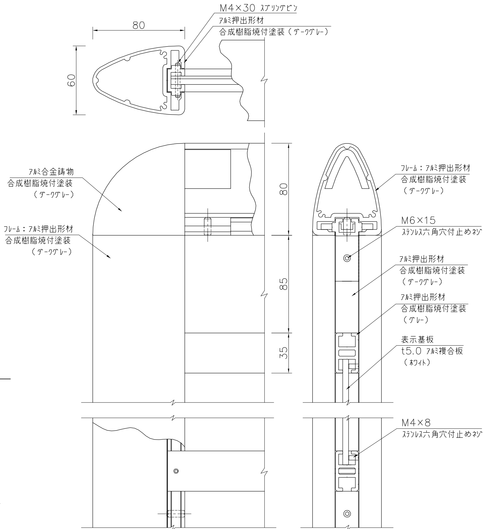
詳細図 S=1/2
