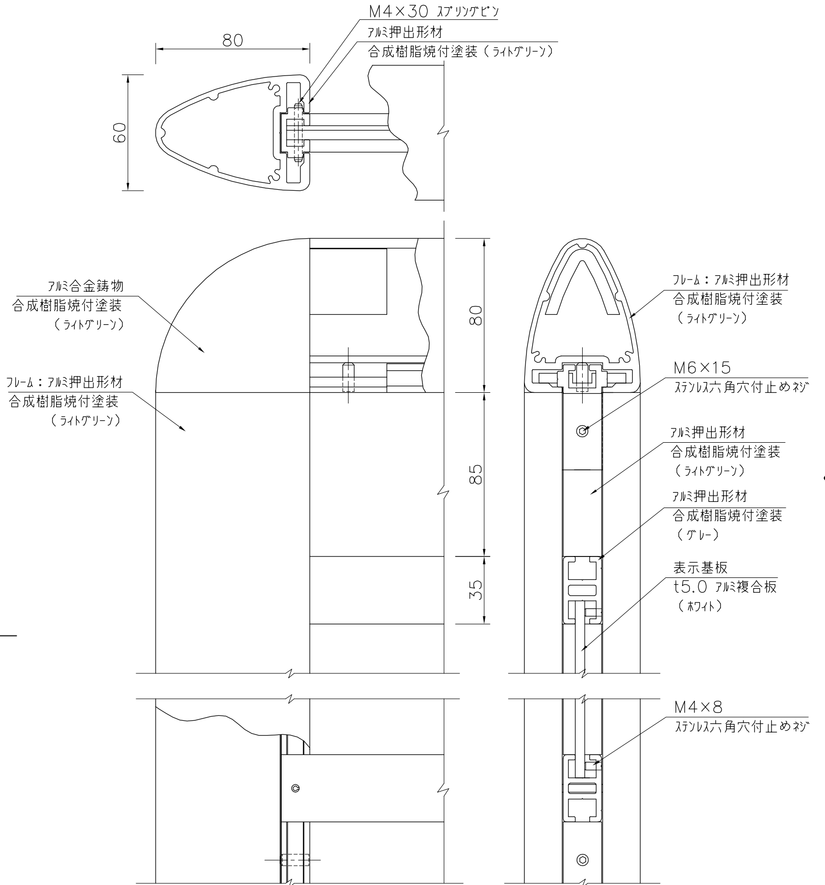
詳細図 S=1/2
