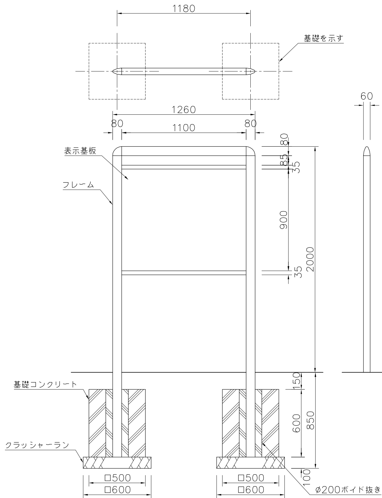
外観図 S=1/20
