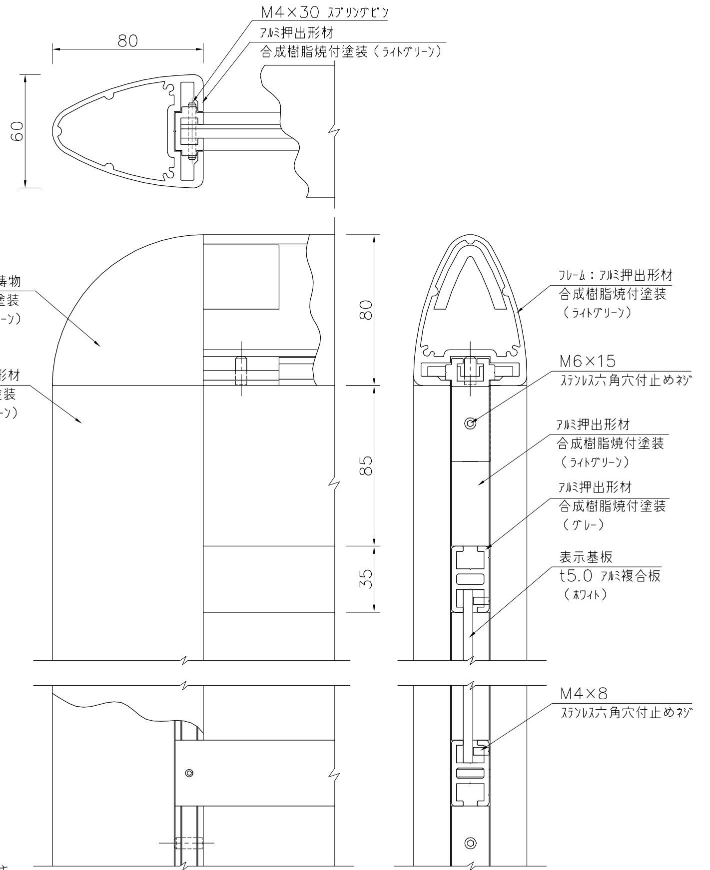
詳細図 S=1/2
