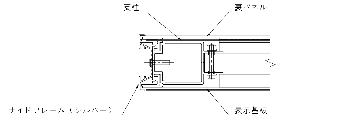
A部断面詳細図 S=1/3
