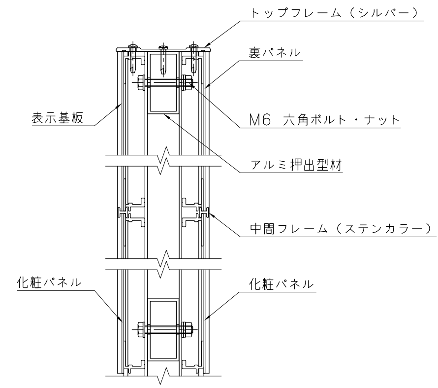
B部断面詳細図 S=1/3
