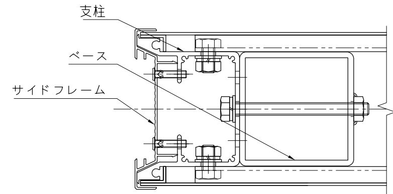
A部断面詳細図 S=1/3
