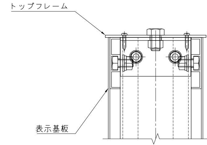
B部断面部分詳細図 S=1/3
