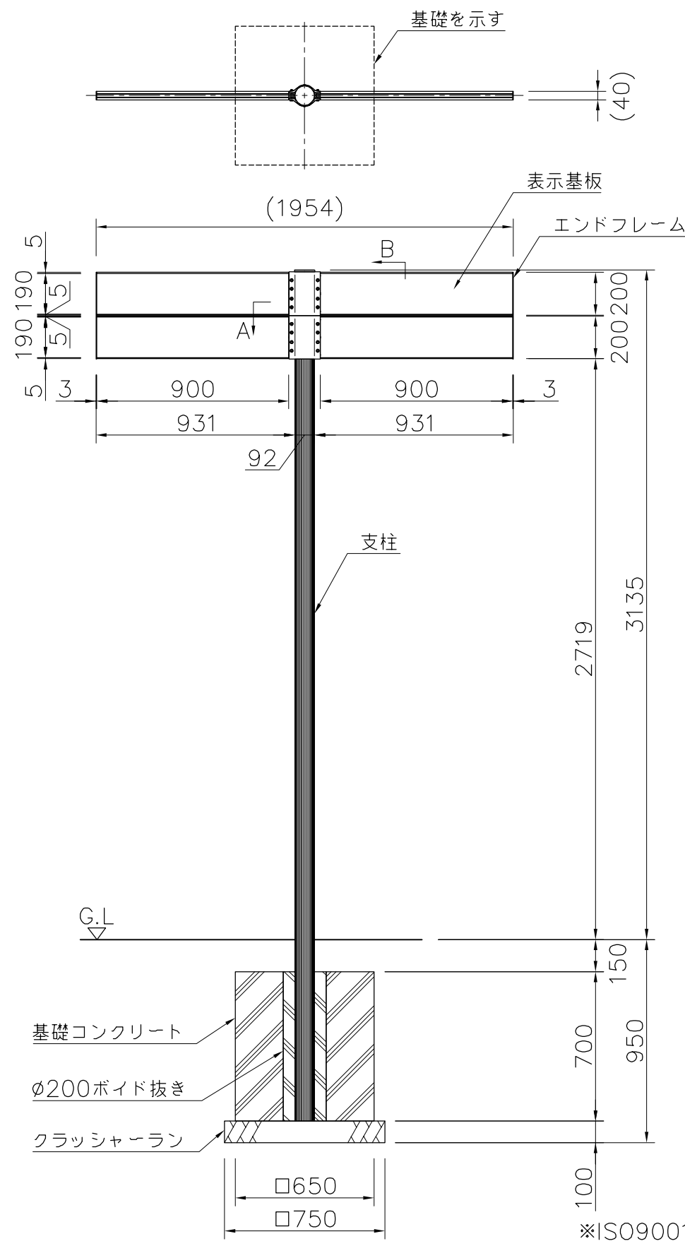
外観図 S=1/25
