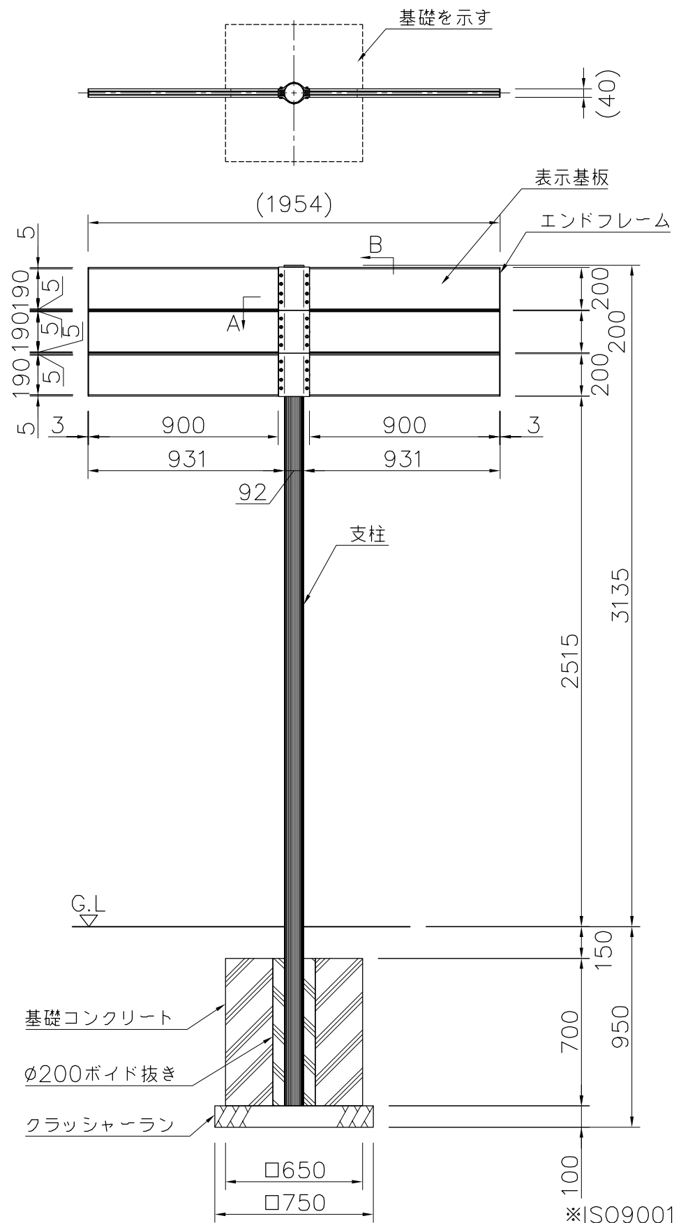
外観図 S=1/25
