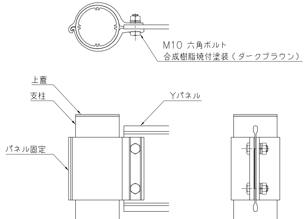
詳細図 S=1/4
