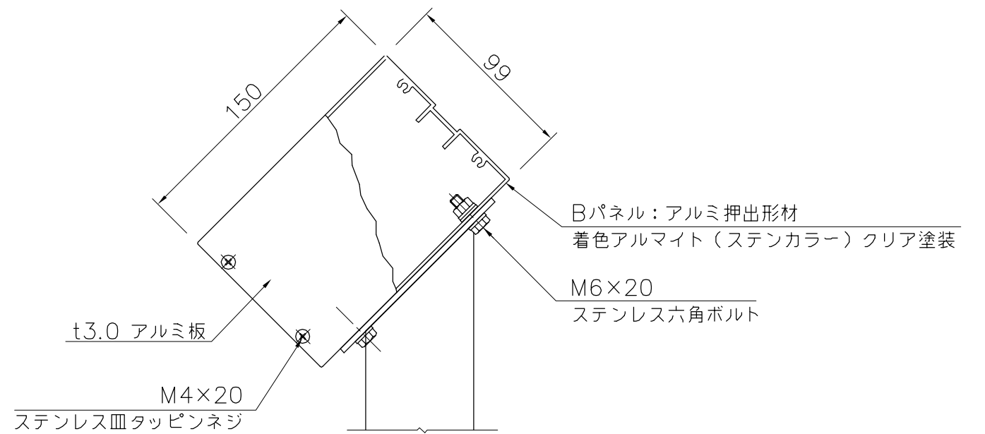
詳細図 S=1/3
