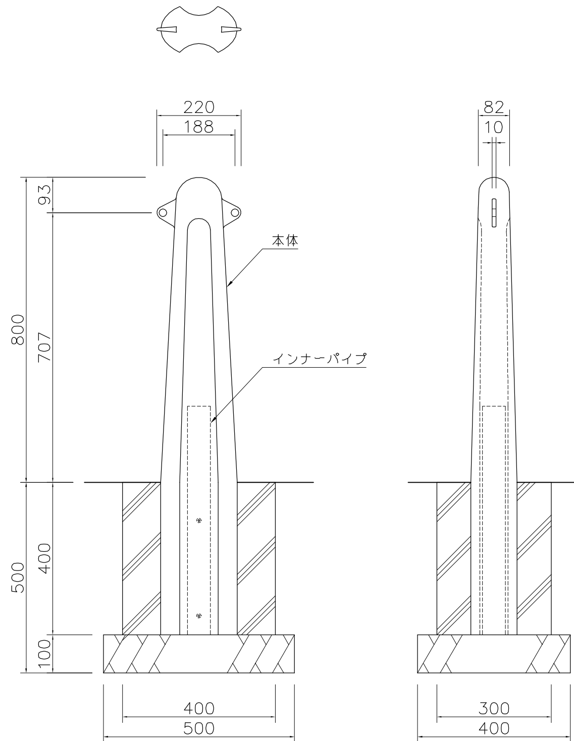
外観図 S=1/10
