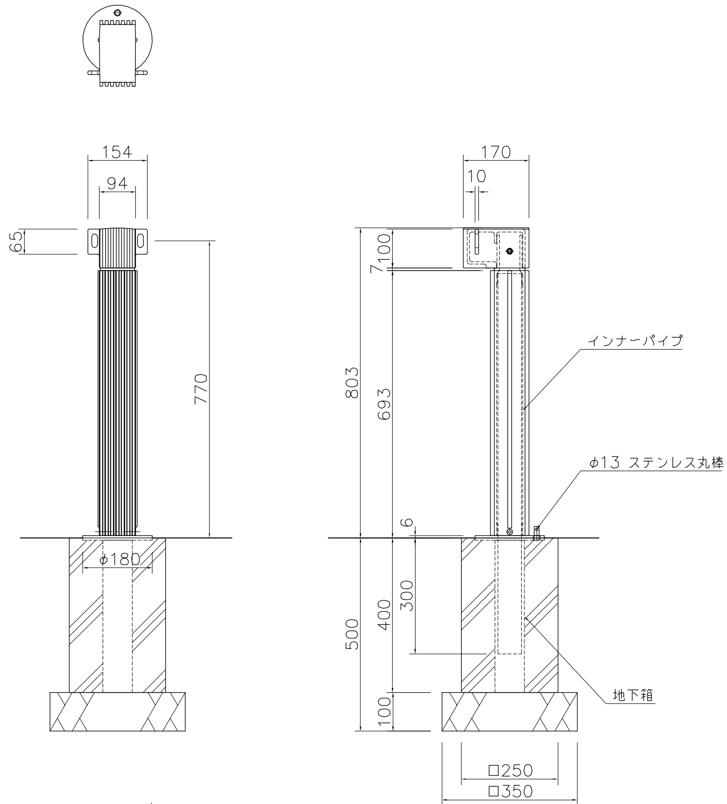
外観図 S=1/10
